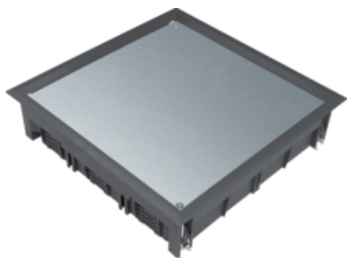
tehalit.VE-EE Pokrywa pełna VDQ12 244x244 wykładzina 12mm czarny PA
