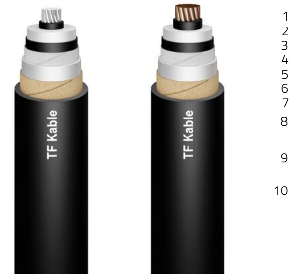
Rys. 3: KABLE ELEKTROENERGETYCZNE WN o izolacji XLPE i POWŁOKĄ ołowianą
